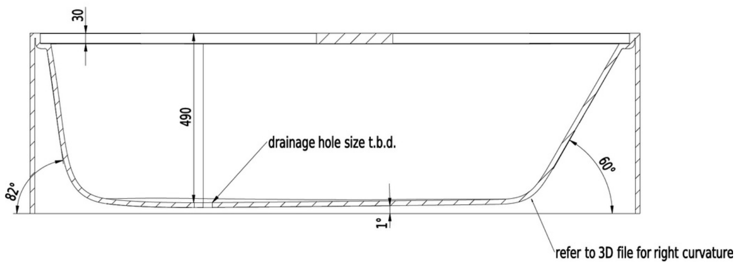
SECTION A-A
